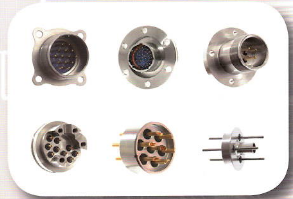
MIL-C-26482 Connectoren
